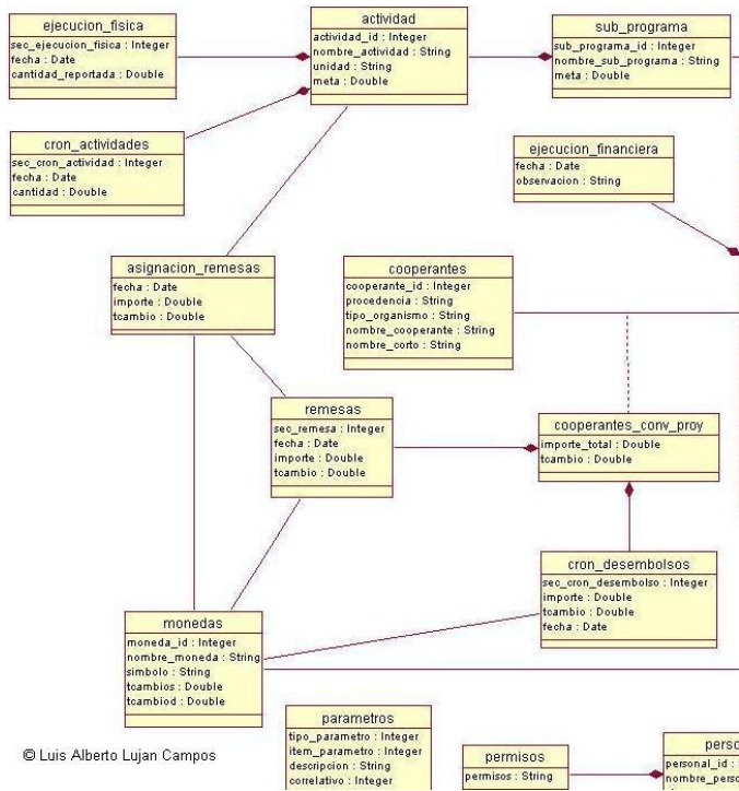
Figura 4: Diagrama de clases de objetos (parte 1).
