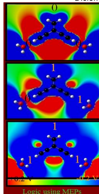
Figura 2. Compuertas lógicas moleculares basadas en el potencial electrostático molecular. El gráfico muestra a una compuerta OR que está compuesta por un 1,1-diethynylethene y dos moléculas de agua (input).
