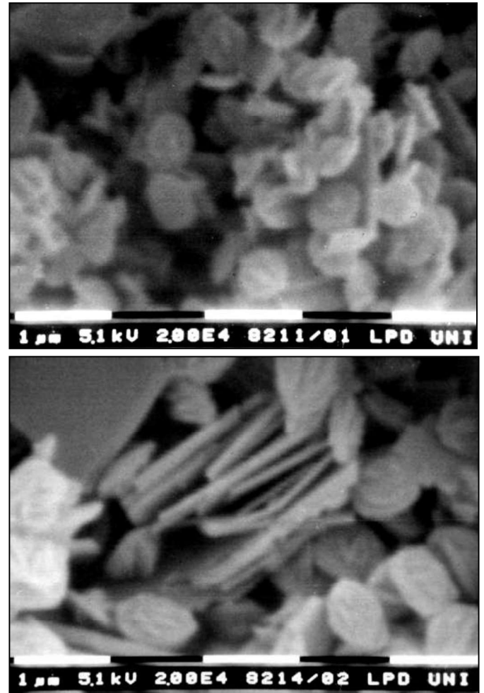
Figura 2: Micrografías MEB de nanopartículas de óxido de cobre obtenidas por radiación gamma a las dosis de 8 y 25 kGy
