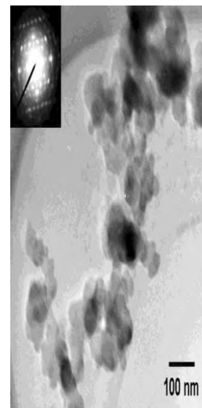
Figura 3: Micrografías MET de partículas de CuO impregnadas en tejidos de algodón.
