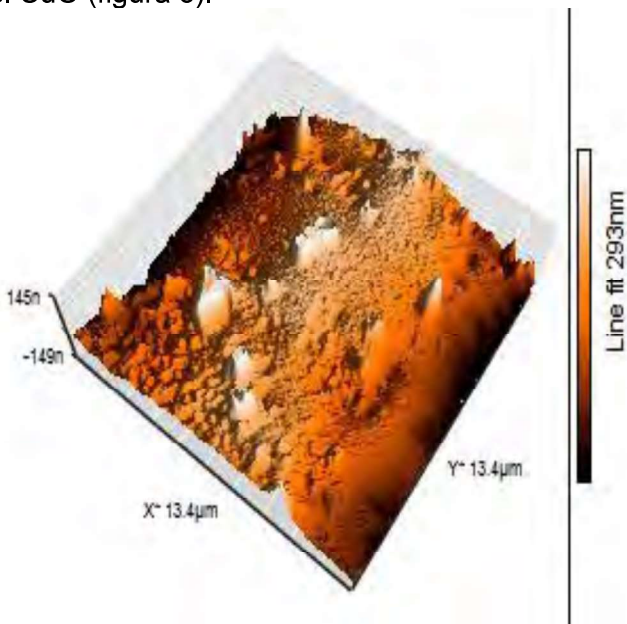
Figura 5: Análisis por AFM, se aprecia la naturaleza microestructurada del material obtenido por técnica sonoquímica.
