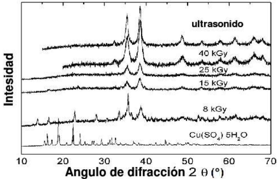
Figura 4: Patrones de difracción de rayos X correspondientes al \text{CuO} y \text{Cu}_4\text{SO}_4(\text{OH})_6 obtenidos por ultrasonido y radiación gamma a las dosis de 8, 15, 25 y 40kGy.
