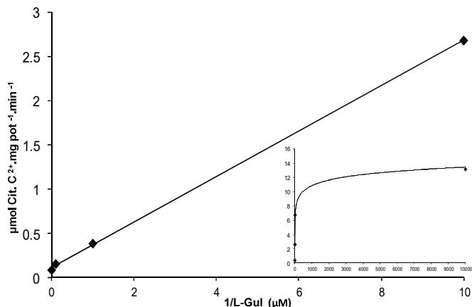
Fig 3. Lineweaver-Burk plots de la actividad catalíticade L-GuLDH en función a la concentración de L-Gulonono-1,4-lactona
