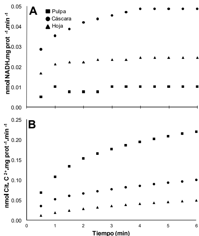
Fig 1. Actividad catalítica de L-GalDH (A) y L-GuLDH (B) en hoja, pulpa y cáscara de M. dubia "camu-camu"
