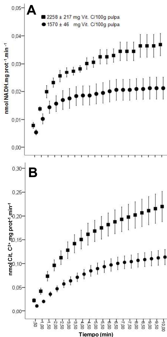
Fig 2. Comparación de la actividad catalítica de L-GalDH (A) y L-GuLDH (B) en pulpa de frutos de M. dubia "camu-camu" que presentan alto y bajo contenido de vitamina C
