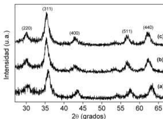
Figura 6: Difragtogramas de rayos-X de la magnetita a) pura e funcionalizada con ácidos grasos de b) Mauritia flexuosa L. c) Copaifera longsdorfii .
