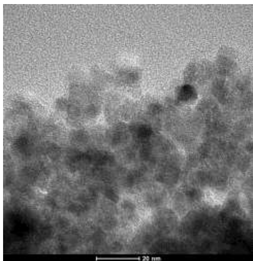
Figura 5: Imagen MET de nanopartículas de Fe_3O_4 preparado con el tercer método recubierta con oro funcionalizado con ácidos grasos de Mauritia flexuosa L.
